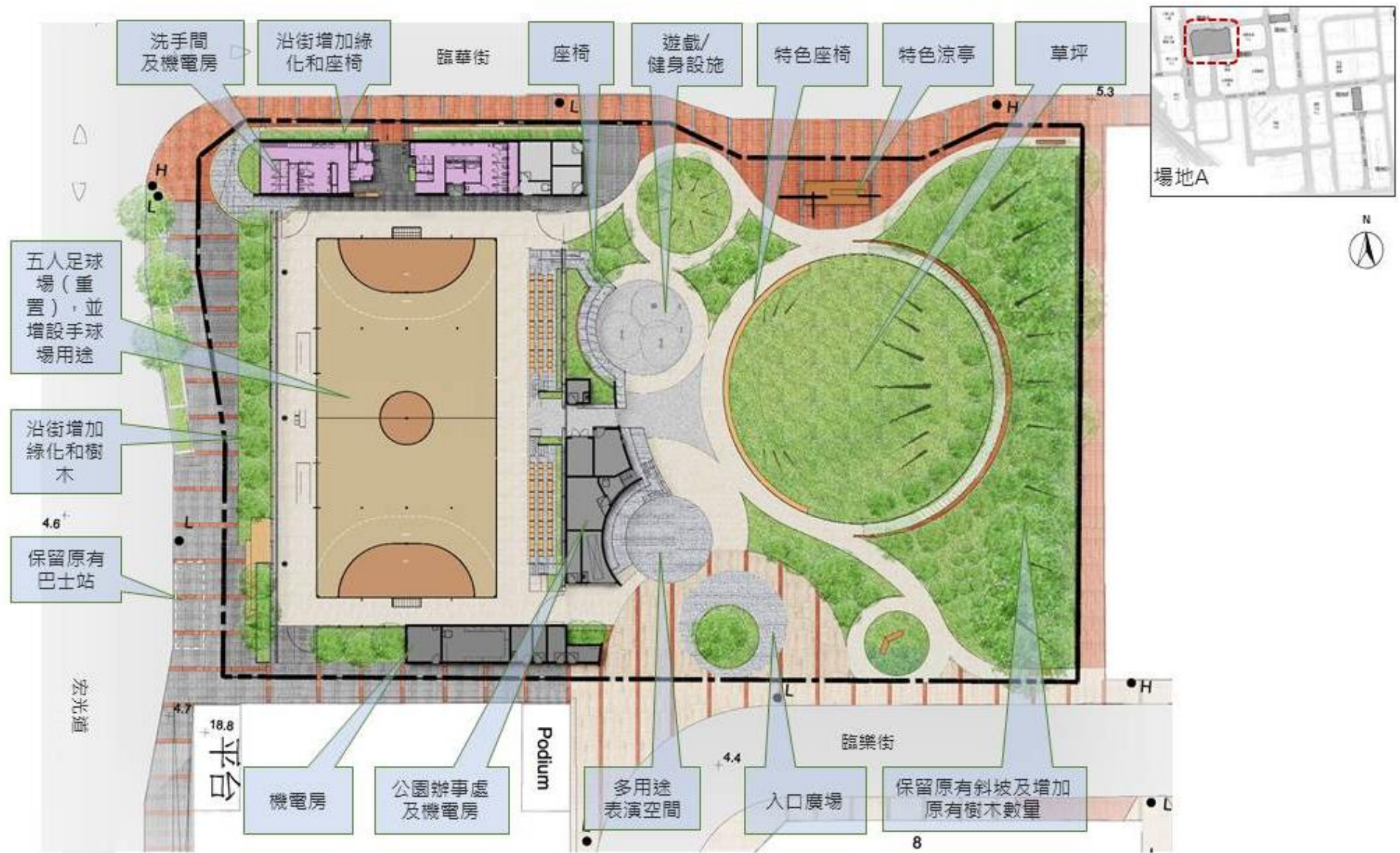
附件二 - 「臨華街遊樂場及其鄰近範圍改善工程」的設計概念圖
